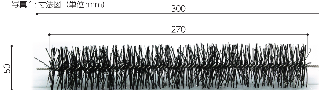
写真1: 寸法図 (単位:mm)
