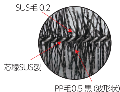
写真2: ブラシ拡大写真
